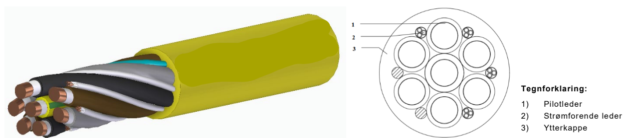
Figur 7 – Fleksibel kabel med pilotledere
