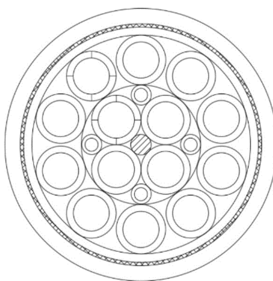
Figur 6 – Eksempel på kabel med fire parallelle ledere per fase og fire pilotledere
