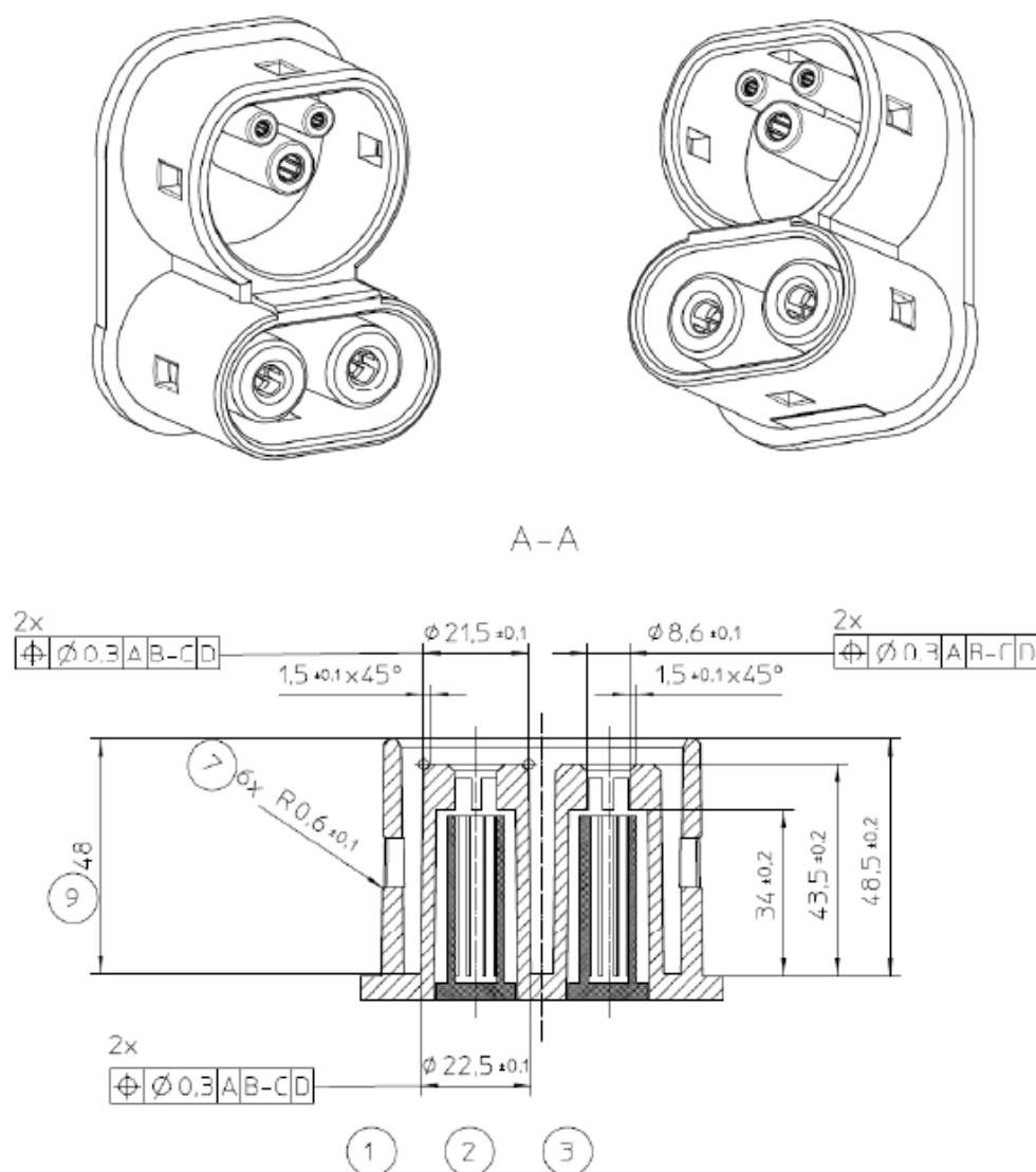
Figur 10 – Dimensjonsblad for DC-kontakten i henhold til EN IEC 62196-3:2022 Konfigurasjon FF (CCS2)
