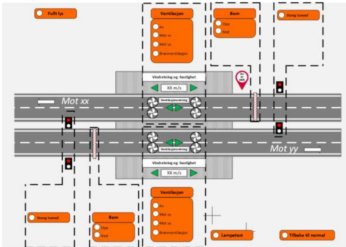
Figur 14.5.1.2 Nødstyrepanel to løp
